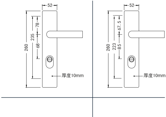
不锈钢防盗把手 产品型号：81202-68/85 FDS 门边距：60mm 中心距：68mm/85mm 产品材质：不锈钢 表面处理：不锈钢拉丝 拉丝锆金 黑色 枪灰
