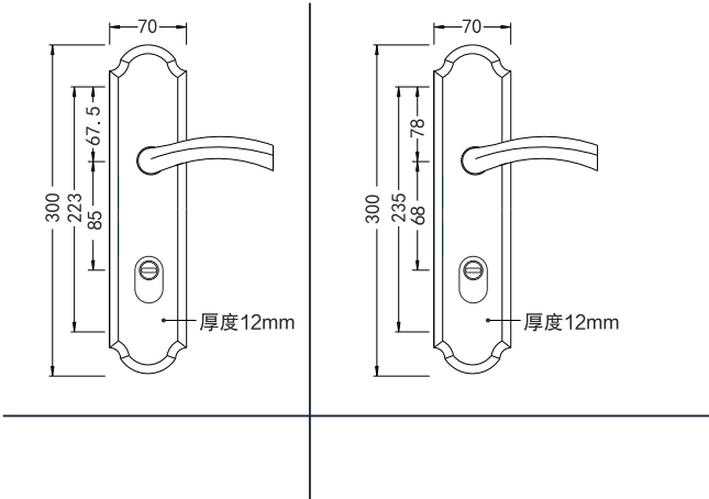
不锈钢防盗把手 产品型号：88347-68/85 FDS 门边距：60mm 中心距：68mm/85mm 产品材质：不锈钢 表面处理：不锈钢拉丝 拉丝锆金 黑色 枪灰
