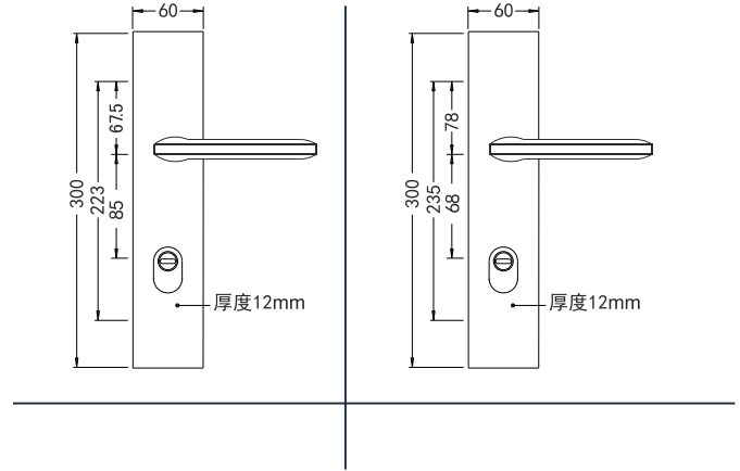
不锈钢防盗把手 产品型号：87755-68/85 FDS 门 边 距：60mm 中 心 距：68mm/85mm 产品材质：不锈钢 表面处理：不锈钢拉丝 拉丝锆金 黑色 枪灰
