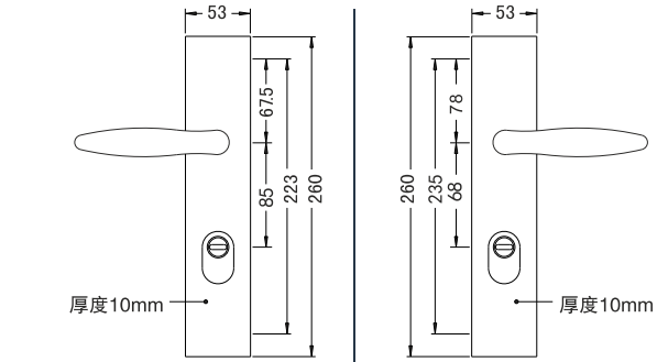
不锈钢防盗把手 产品型号：82744-68/85 FDS 门 边 距：60mm 中 心 距：68mm/85mm 产品材质：不锈钢 表面处理：不锈钢拉丝 拉丝锆金 黑色 枪灰
