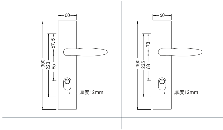
不锈钢防盗把手 产品型号：87744-68/85 FDS 门 边 距：60mm 中 心 距：68mm/85mm 产品材质：不锈钢 表面处理：不锈钢拉丝 拉丝锆金 黑色 枪灰
