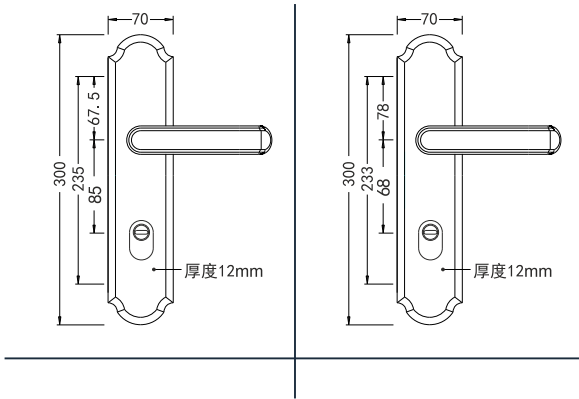
不锈钢防盗把手 产品型号：88373-68/85 FDS 门边距：60mm 中心距：68mm/85mm 产品材质：不锈钢 表面处理：不锈钢拉丝 拉丝锆金 黑色 枪灰
