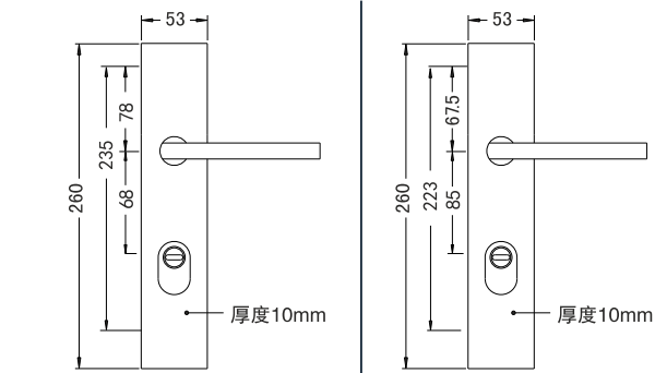
不锈钢防盗把手 产品型号：82754-68/85 FDS 门 边 距：60mm 中 心 距：68mm/85mm 产品材质：不锈钢 表面处理：不锈钢拉丝 拉丝锆金 黑色 枪灰
