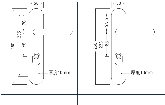
不锈钢防盗把手 产品型号：81103-68/85 FDS 门边距：60mm 中心距：68mm/85mm 产品材质：不锈钢 表面处理：不锈钢拉丝 拉丝锆金 黑色 枪灰
