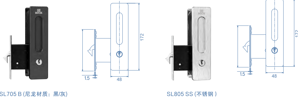
SL705 B (尼龙材质: 黑/灰)
