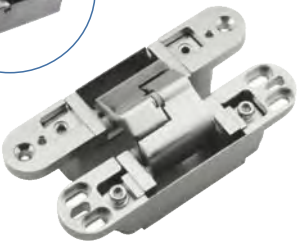
型号：RKB005(不分左右) 尺寸：28X135X140mm
