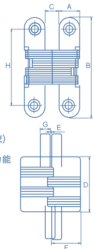
型号：RKA005 尺寸：16X70X11mm
