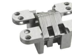
型号：RKC002T 尺寸：28X118X22mm 说明：不锈钢叠片式暗铰链
