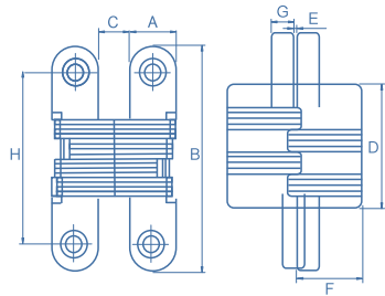
型号：RKC001T~RKC007T (不锈钢消音暗铰链-可选内置尼龙片，具有消音功能)
