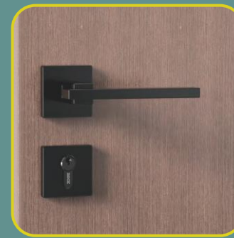
铝合金: 60445-F 铝氧化黑色 不锈钢: 80445-F 不锈钢黑色 锌合金: 90445-F 锌合金黑色
